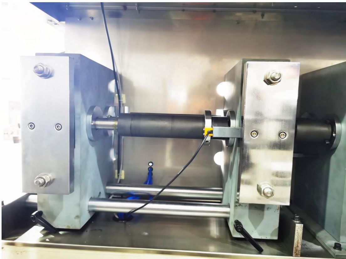
可调式挂膜机构调节方便 适用多种规格
