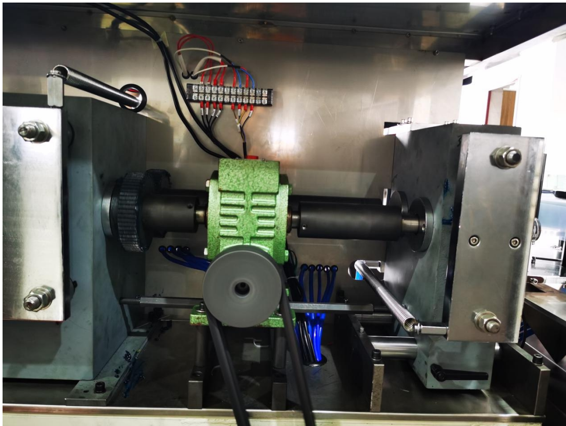
产品驱动机构
