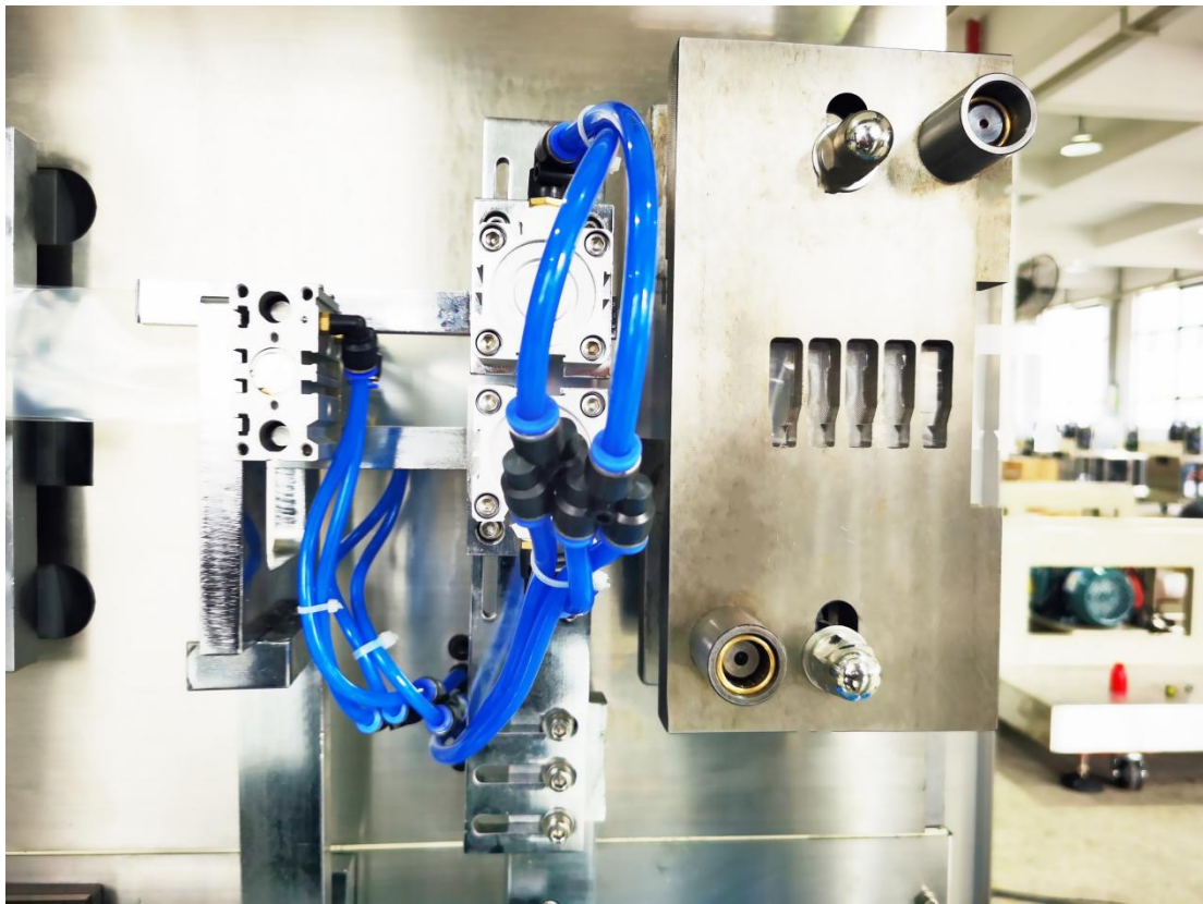
多列产品模切出料机构 速度更快
